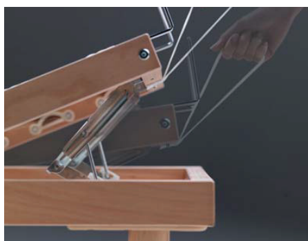
механизм ручного подъема
